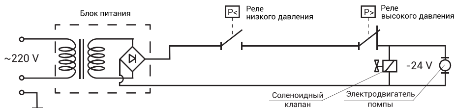
Рис. 14. Электрическая схема фильтра Accord RO.
